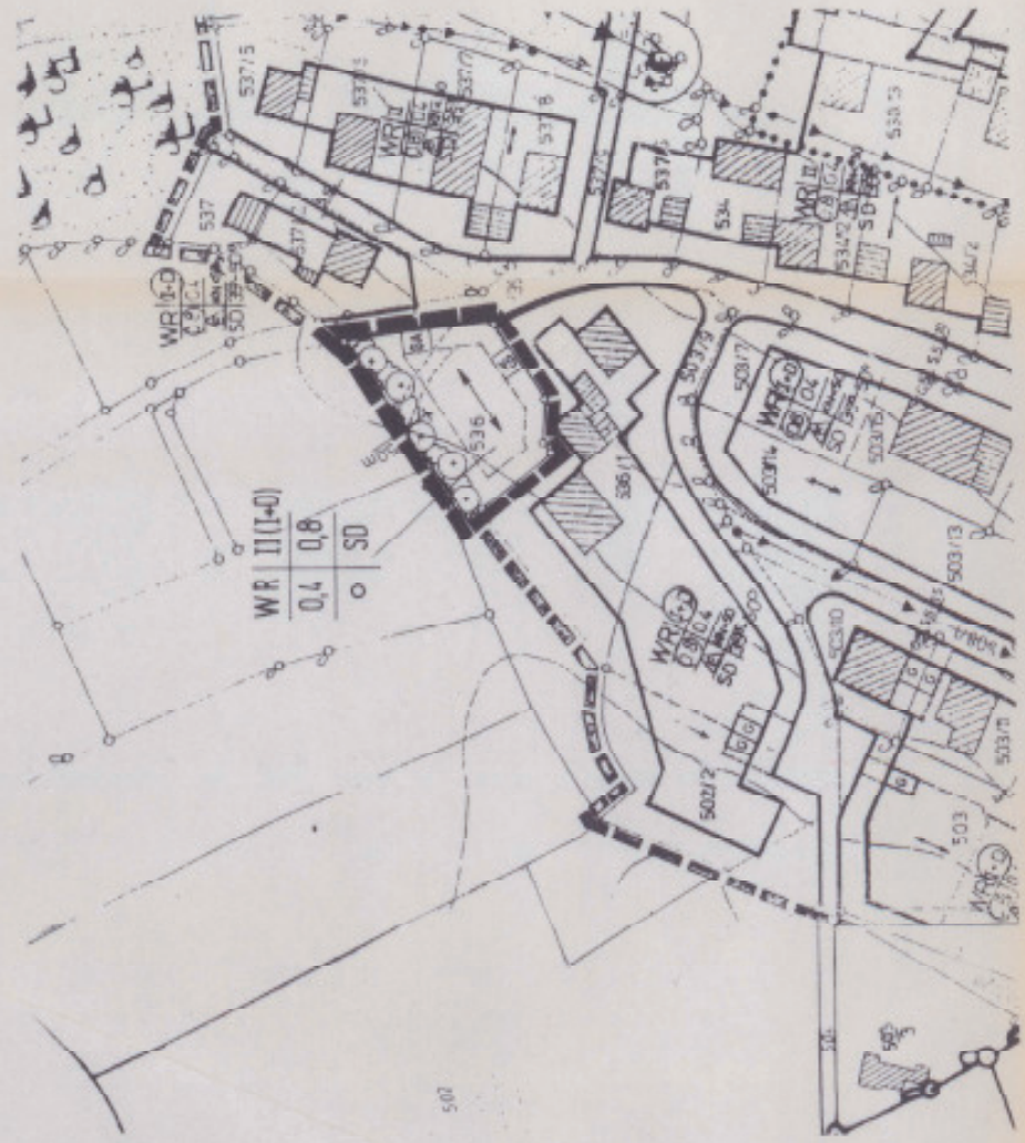
AUSSCHNITT AUS DEM RECHTSKRÄFTIGEN BEBAUUNGSPLAN NW3 VON 31.6.1994
